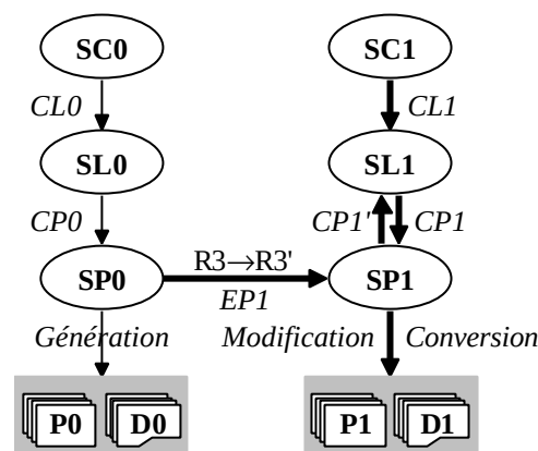
Figure 11 - Propagation vers l'aval des modifications déduites de R3 ® R3' et reconstruction de CP1
