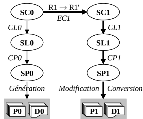
Figure 7 - Propagation vers l'aval des modifications déduites de R1 ® R1'.
