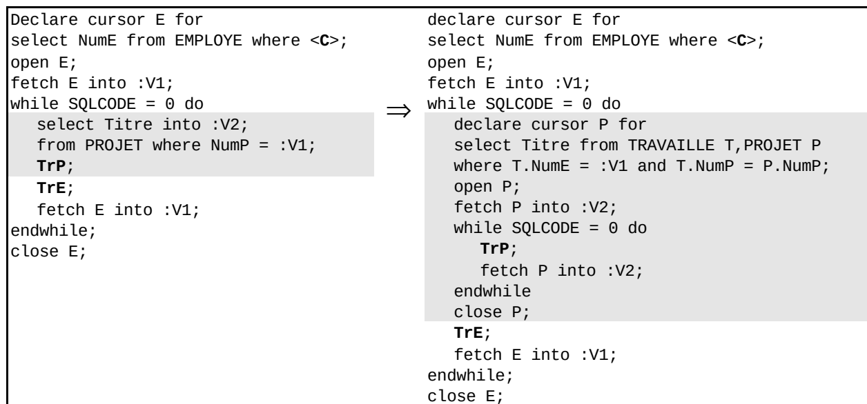
Figure 9 - Impact sur un programme de la modification de la figure 8.
