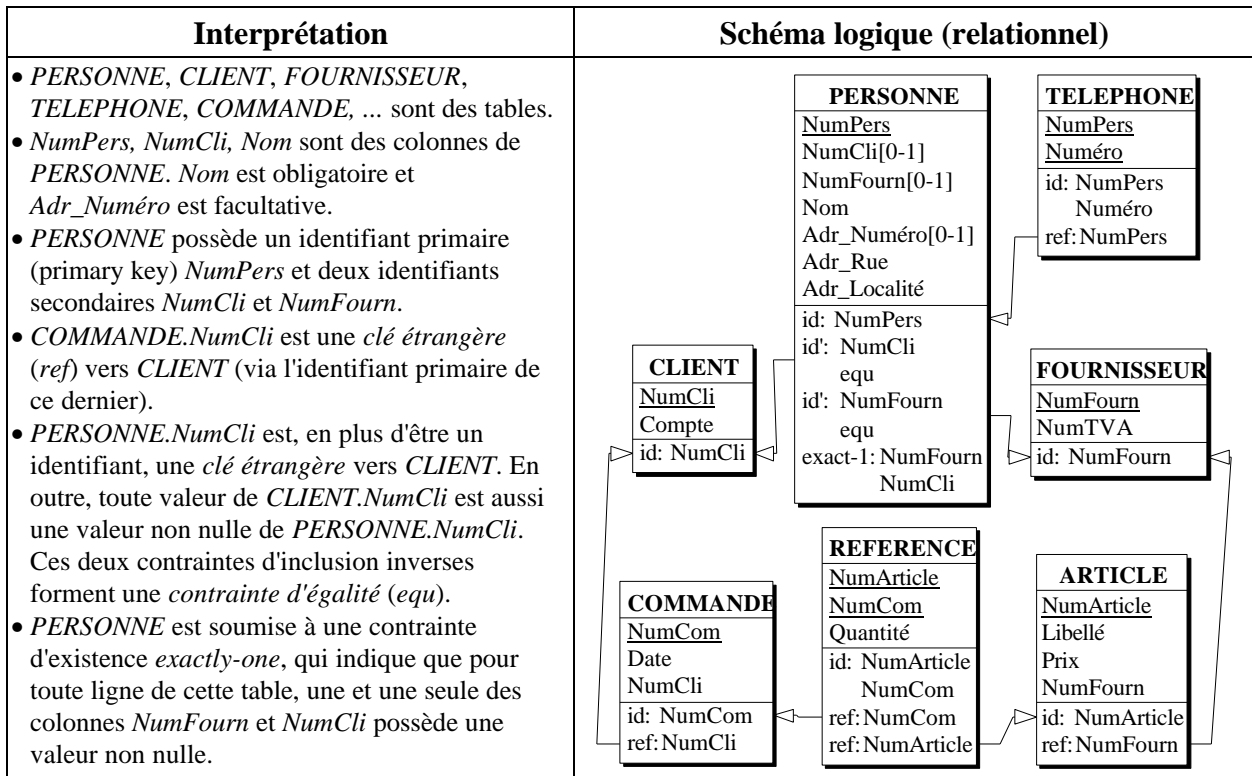
Figure 3 - Vue graphique et interprétation d'un schéma logique relationnel.
